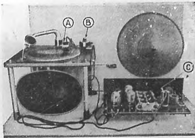
Un reproductor eléctrico conectado y listo para funcionar. Los únicos accesorios que se necesitan son: Un acumulador de seis voltios y un altoparlante. Si el reproductor se emplea en combinación con un amplificador audíofono, el acumulador de seis voltios debe reemplazarse con una pila seca de uno y medio voltios.
