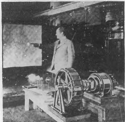
El doctor E. F. W. Alexanderson en su laboratorio, señalando los siete rayos luminosos que se usan en el método propuesto por él para la televisión. En el primer plano se ve el tambor en el que se han instalado los espigas, accionado con el motor que lo hace girar. También puede verse un sistema de lentes, junto con una lámpara de acero.
